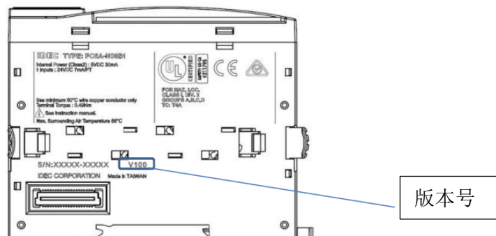
图 2: 数字 I/O 模块硬件版本号
