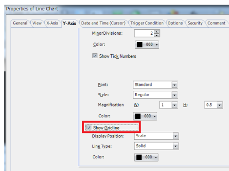
图 2-2：“显示网格线”设置
