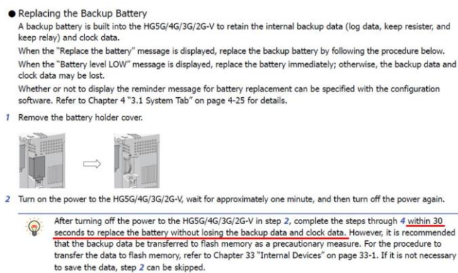
图 4-1. 更换备用电池。(HG5G/4G/3G/2G-V)
