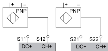
PNP 出力を伴うセンサ / 機器の配線
