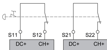
安全柵入力の配線
