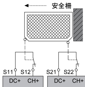
安全柵入力の配線
