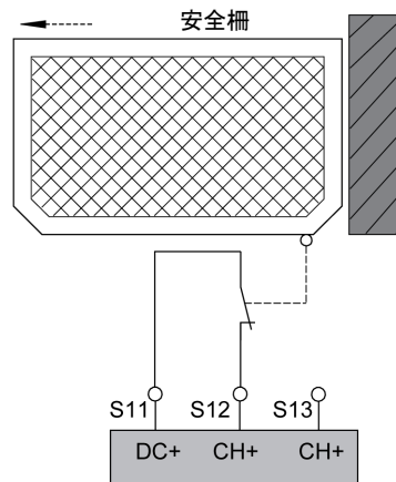
安全柵入力の配線
