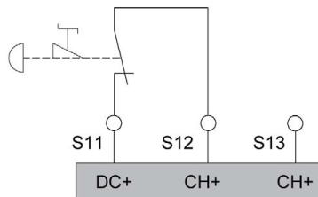
非常停止入力の配線
