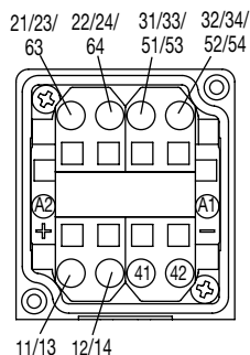
端子排列图
